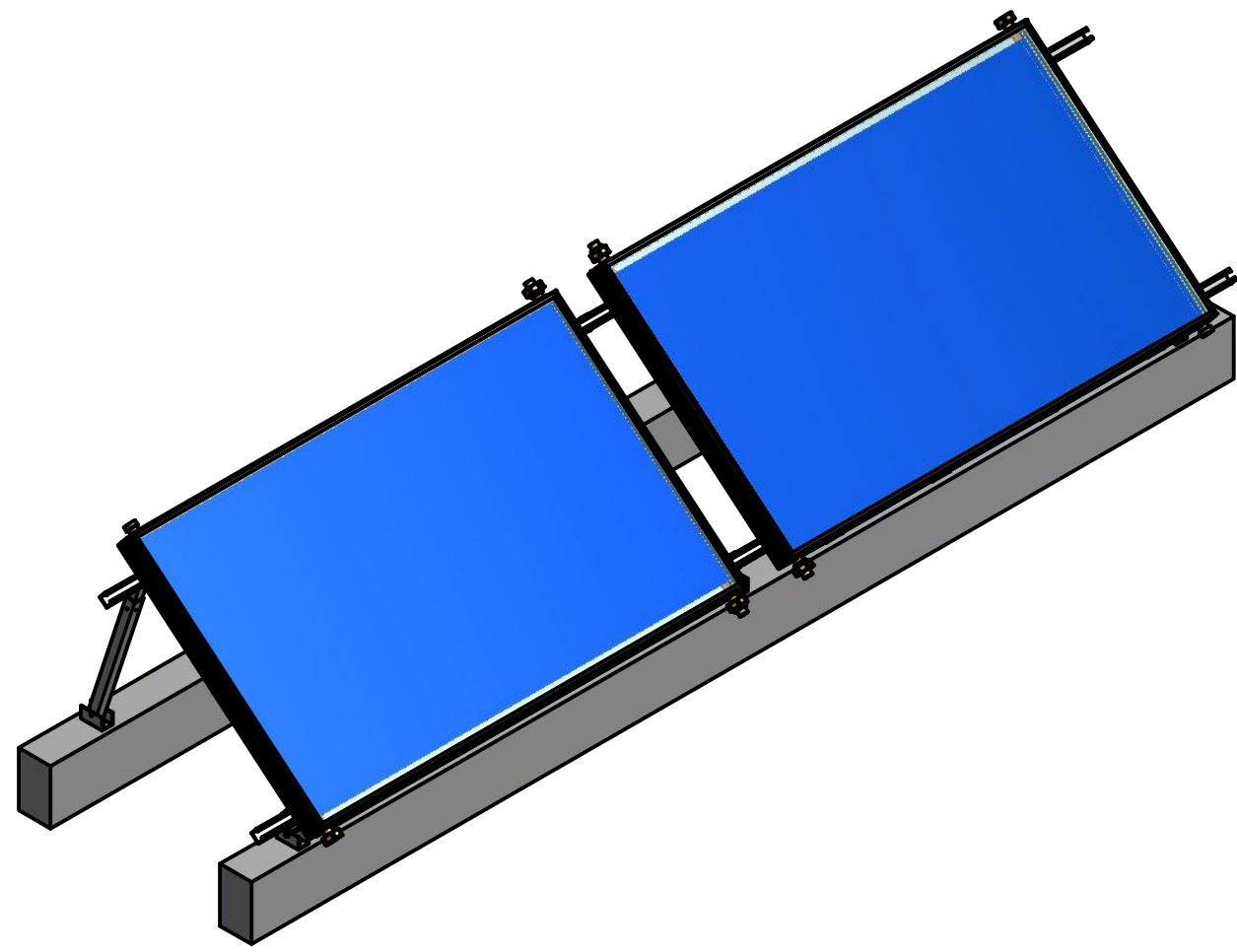
Iso SCALE 1/25
